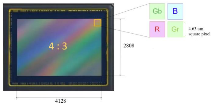
图 1 IMX294 图像传感器及其像素结构
