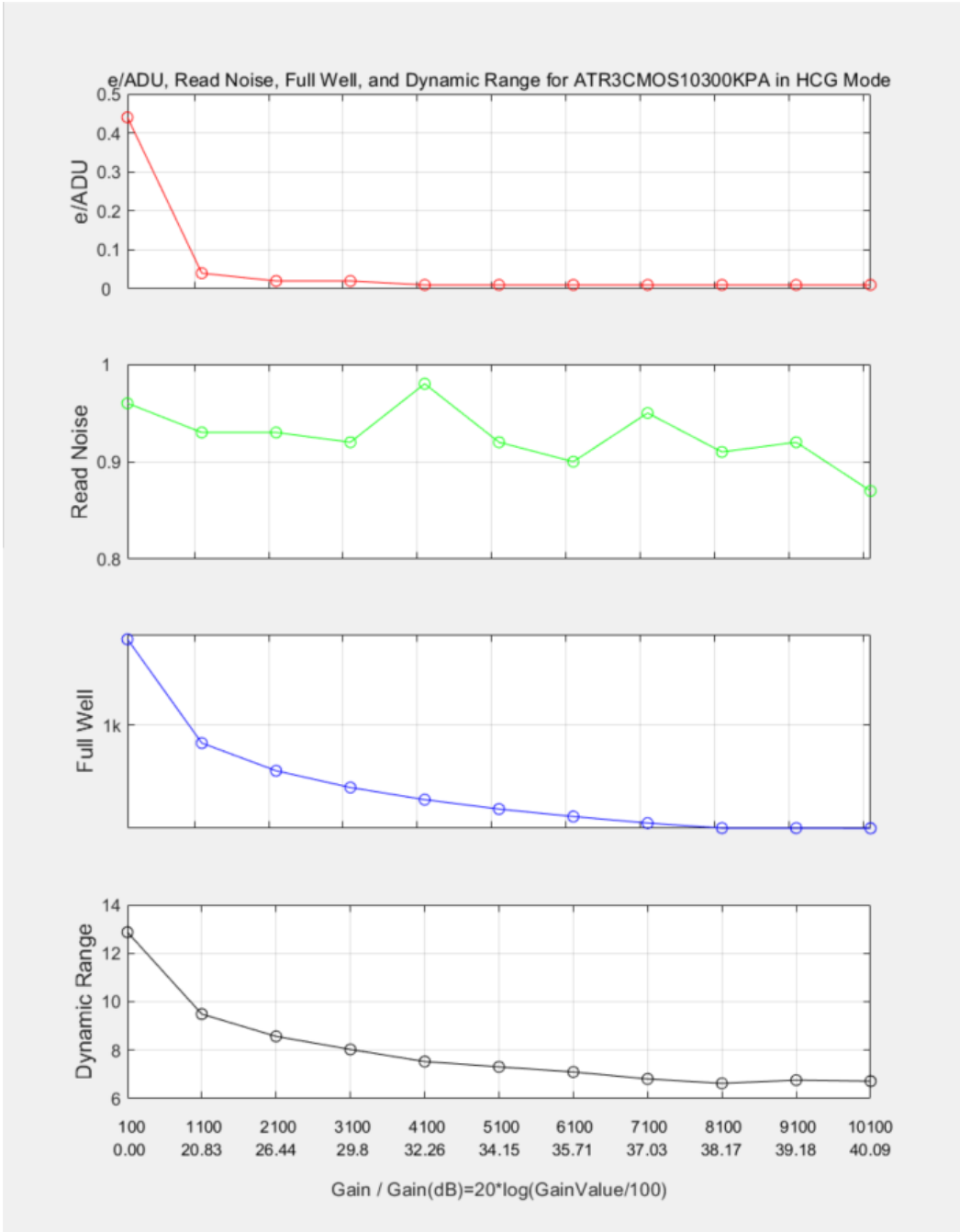
图 6ATR294C 的 e-/ADU、读出噪声、满阱电荷和动态范围
