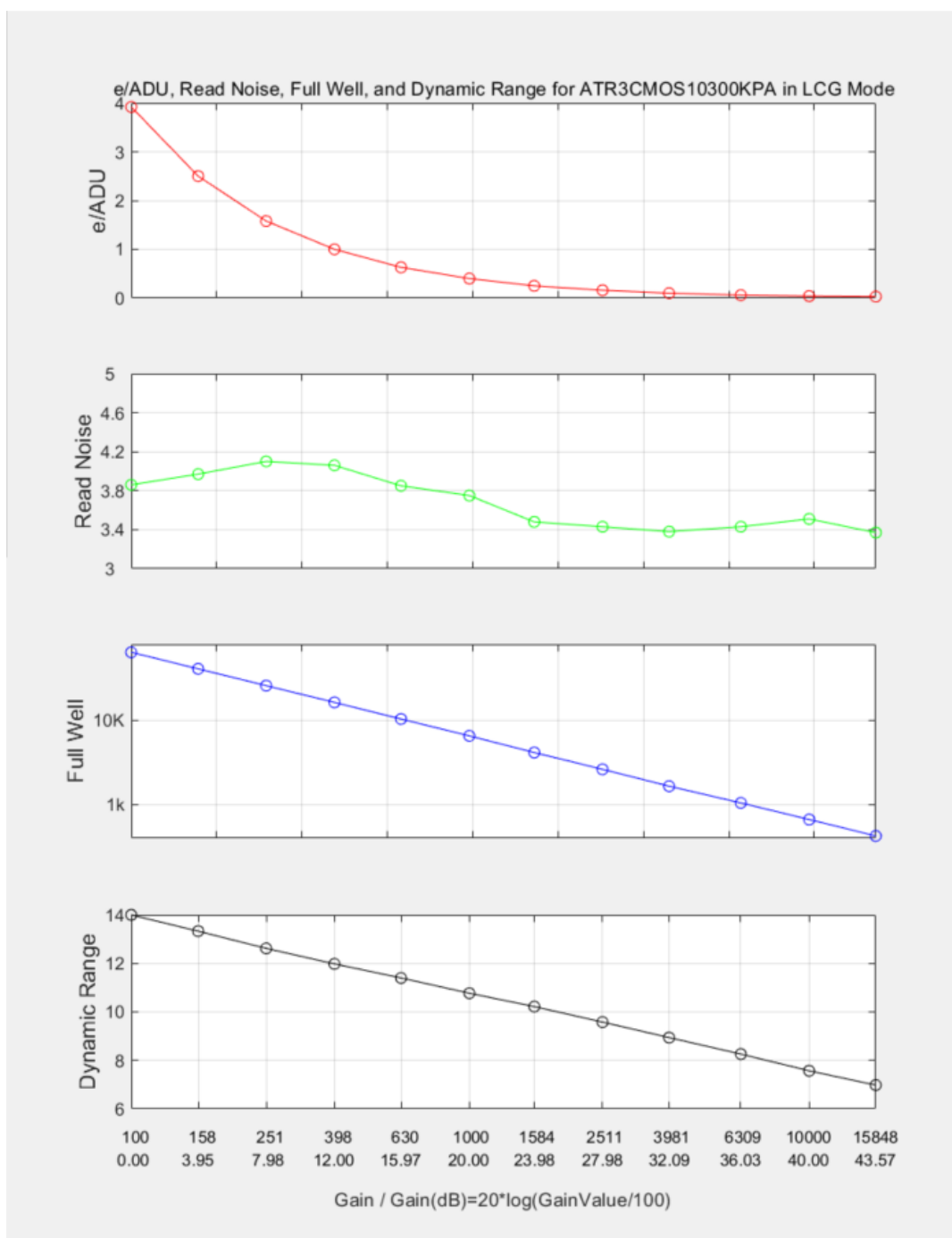
图 5 ATR294C 的 e-/ADU、读出噪声、满阱电荷和动态范围
