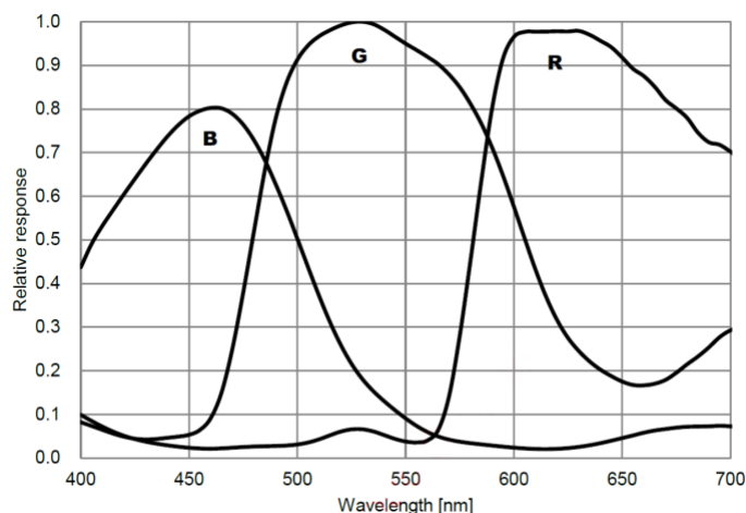
图 2 IMX294 光谱灵敏度特性
