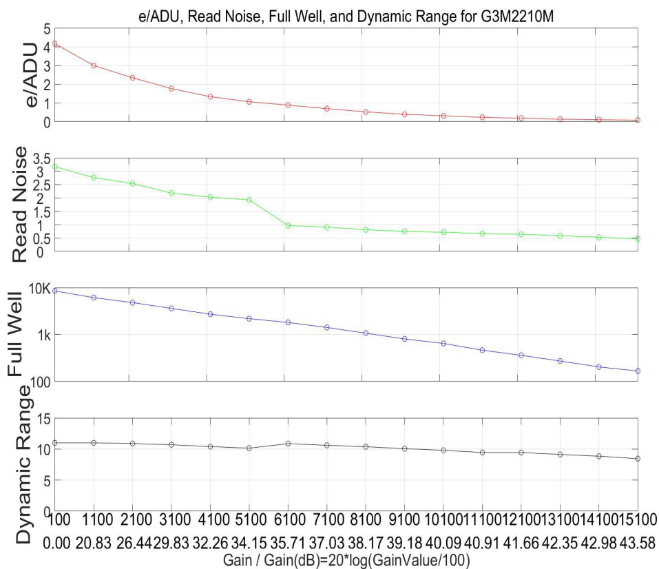
图 2 G3M2210M 的 e-/ADU、读取噪声、满阱和动态范围
