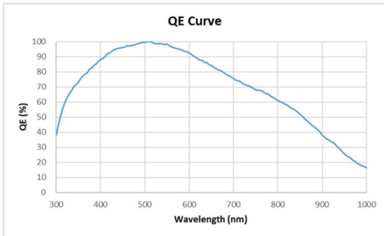
图 1 SC2210 光谱灵敏度特性
