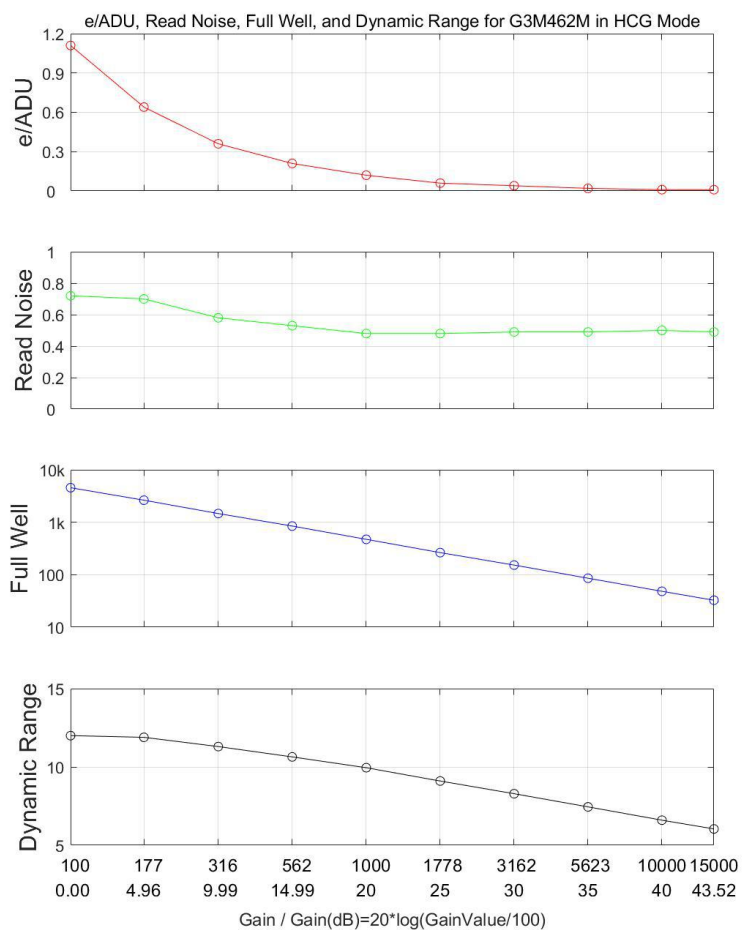
图 3 G3M462M 的 e-/ADU、读取噪声、满阱和动态范围
