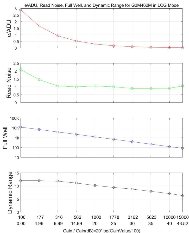
图 2 G3M462M 的 e-/ADU、读取噪声、满阱和动态范围
