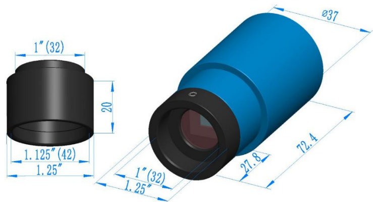
图 2G3M462M 的尺寸和安装座
