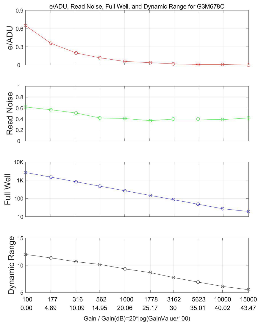
图 3 G3M678C 的 e/ADU、读取噪声、满阱和动态范围
