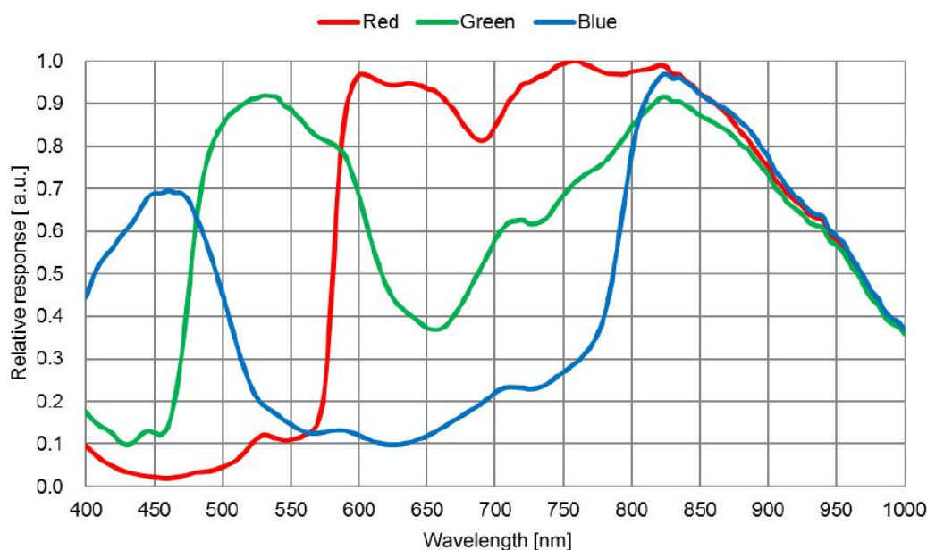
图 1 IMX678 光谱灵敏度特性
