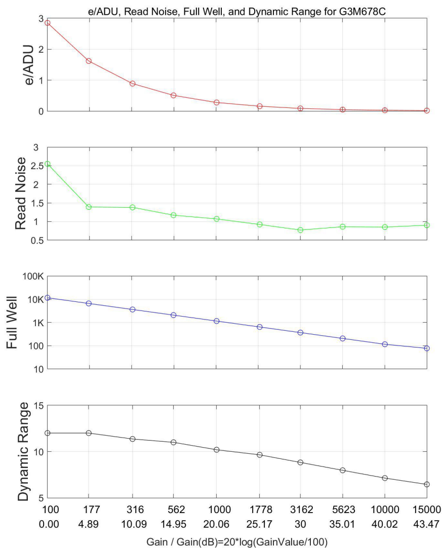
图 2 G3M678C 的 e-/ADU、读取噪声、满阱和动态范围
