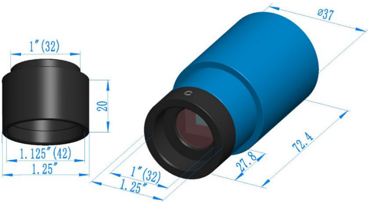
图 2G3M678C 的尺寸和安装座
