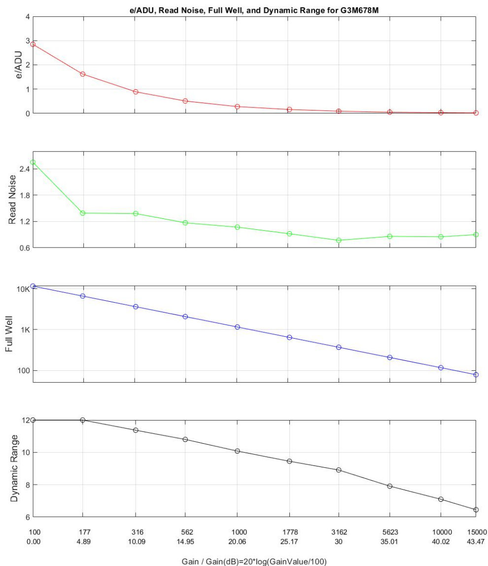
图 4 G3M678M 的 e-/ADU、读取噪声、满阱和动态范围
