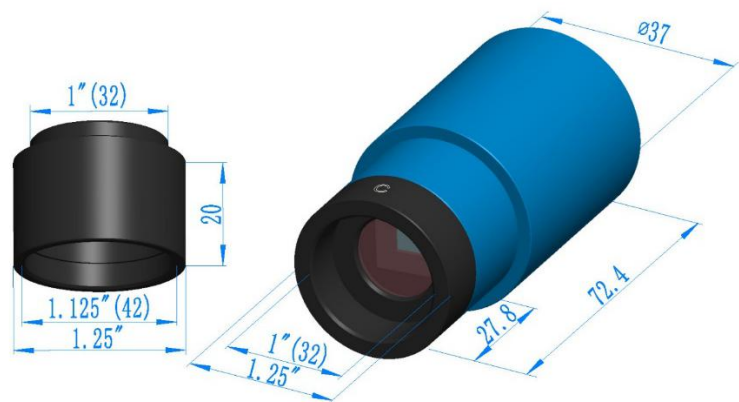
图 2G3M678M 的尺寸和安装座
