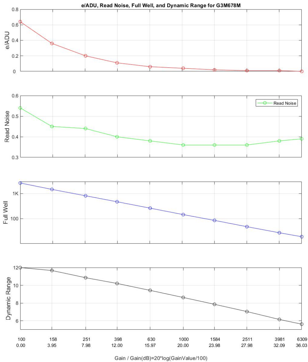
图 5 G3M678M 的 e-/ADU、读取噪声、满阱和动态范围
