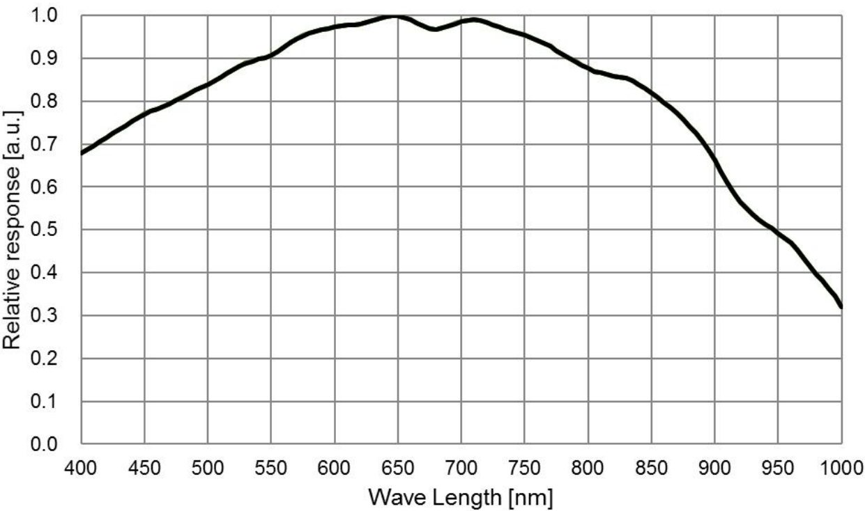
图 1 IMX678 光谱灵敏度特性
